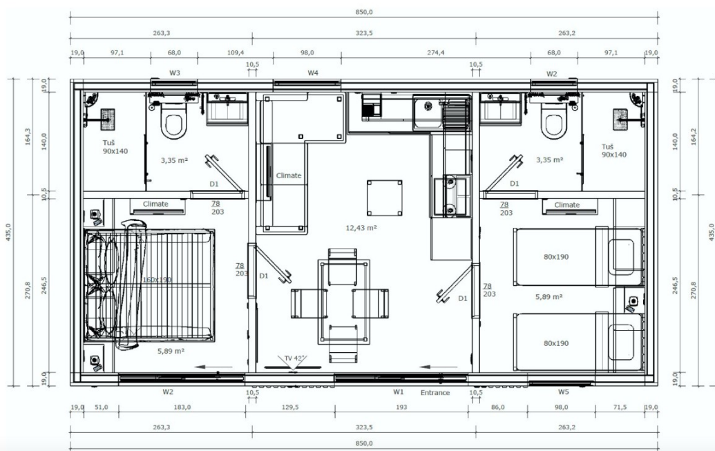
Tlocrt mobilne kuće Leona 36 CAMP
