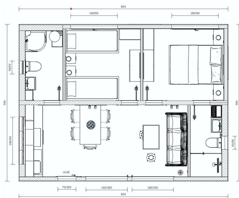
Tlocrt mobilne kuće Leona 48
