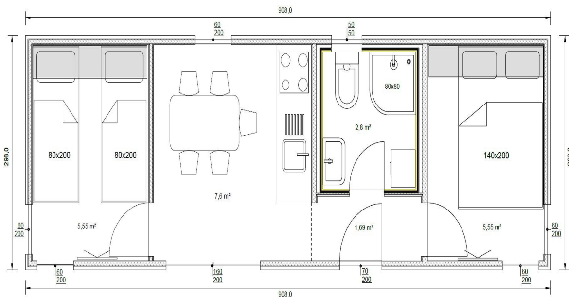
Tlocrt mobilne kuće Leona 27
